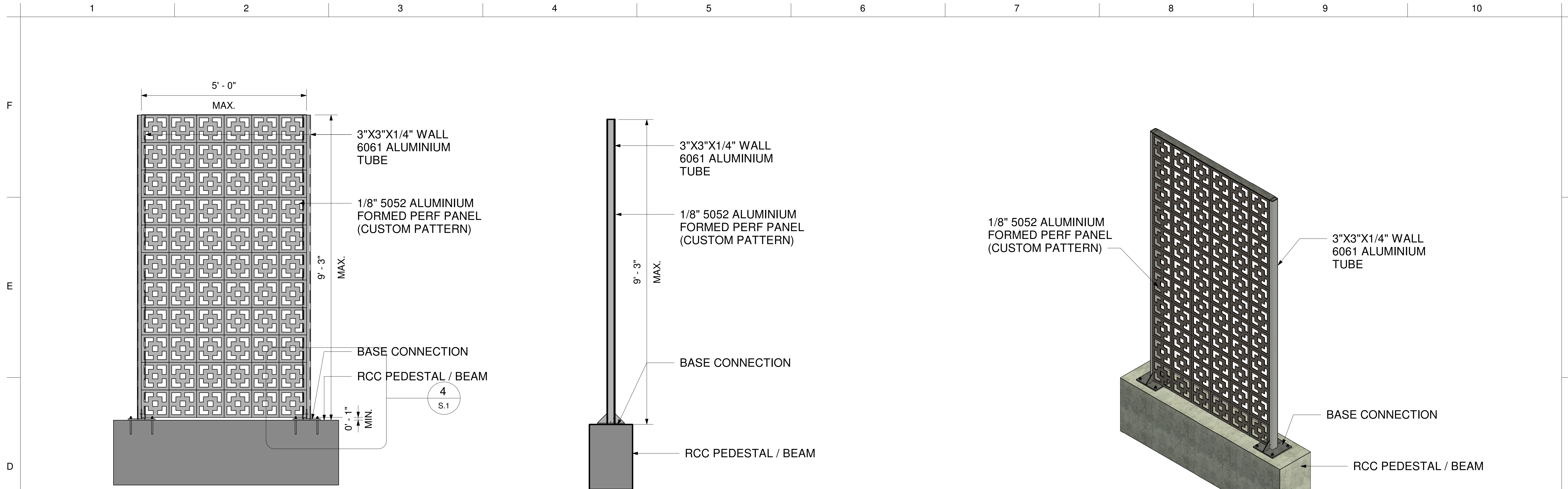
1 ELEVATION 1 : 25
